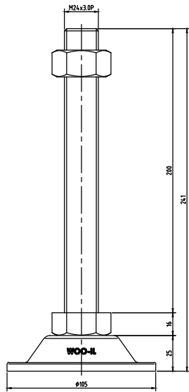
BL105-M24-200
